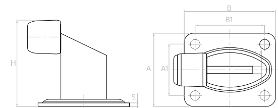
Zderzak zewnętrzny z płytką Gate stopper / Наружный отбойник с креплением / Torstopper mit Platte
