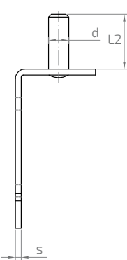
Czop do przykręcenia ozdobny Pin / Петледержатель прикручиваемый / Torband Dorn
