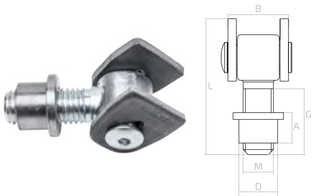
Zawias do wstawiania Welding hinge / Петля приварная / Scharnier zum Einschweißen
