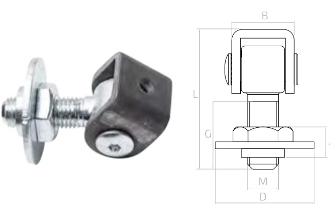
Zawias regulowany do wstawiania Adjustable welding hinge / Регулируемая петля приварная / Verstellbares Scharnier zum Einschweißen
