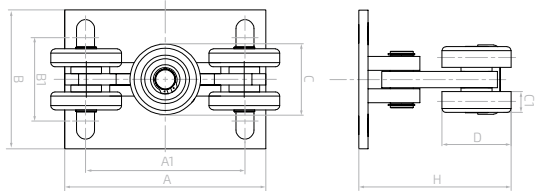
Wózek jezdny 5 rolkowy do szyny 6V.068 Cantilever gate carriage / Роликовая каретка / Laufrollenbock
