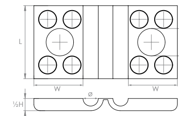
Dystans obejmuj panelowej Spacer for fence brace band / Пластиковый вкладыш для хомута / Doppelschelle-Distanzstück
