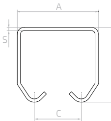
Ceownik do bram podwieszanych Monorail for cantilever gates / Направляющая шина для ворот для подвесной системы / Torprofil
