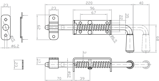
Rygiel ze sprężyną Latch / Щеколда с пружиной / Riegel
