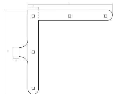
Zawiasy kątowe ozdobne Hinge / Петля / Scharnier
