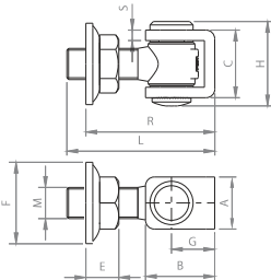
Zawias regulowany Adjustable hinge / Регулируемая петля / Verstellbares Scharnier
