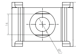
Łącznik ogrodzeń panelowych Mesh fencing connector - green / Хомут / Montageverbinder grün
