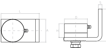
Zawias do bramy dolny, łożyskowy Bottom gate hinge with bearing / Нижний шарнир для ворот / Unteres Torscharnier mit Lagerung
