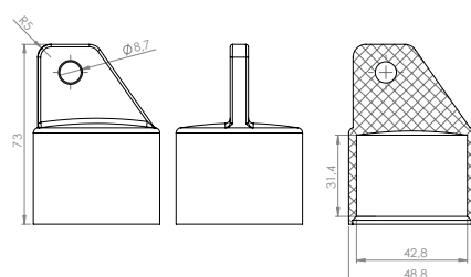
Nasadka słupa podporowego Brace cup / Колпачок подпорного столба / Strebe
