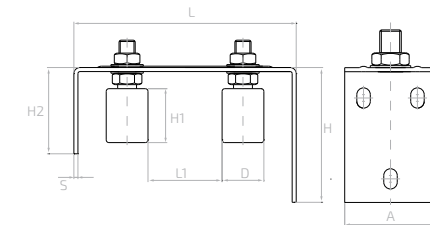
Prowadzenie górne regulowane Adjustable gate guide / Верхние поддерживающие ролики с регулировкой / Laufrollenbock einstellbar
