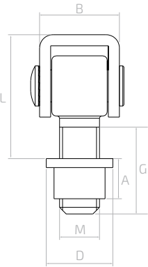
Zawias do spawania Welding hinge / Петля приварная / Scharnier zum Einschweißen
