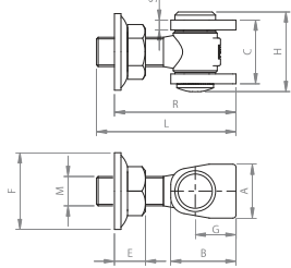
Zawias regulowany Adjustable hinge / Регулируемая петля / Verstellbares Scharnier
