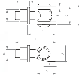
Zawias do spawania Welding hinge / Петля приварная / Scharnier zum Einschweißen
