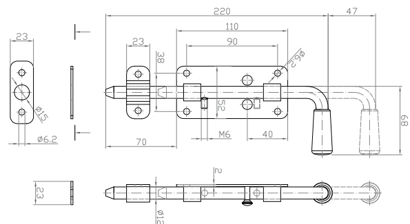
Rygiel Latch / Щеколда / Riegel
