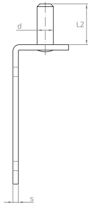
Czop do przykręcenia Pin / Петледержатель прикручиваемый / Torband Dorn
