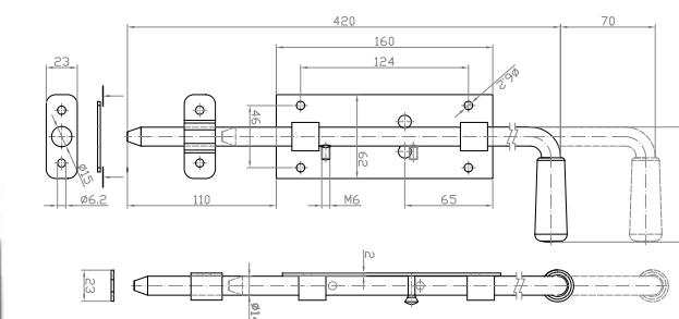
Rygiel wąski Latch / Щеколда / Riegel
