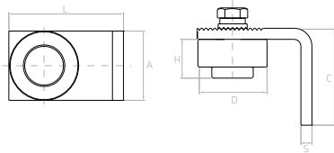
Zawias do bramy górny, łożyskowy Upper gate hinge with bearing / Верхний шарнир для ворот / Oberes Torscharnier mit Lagerung
